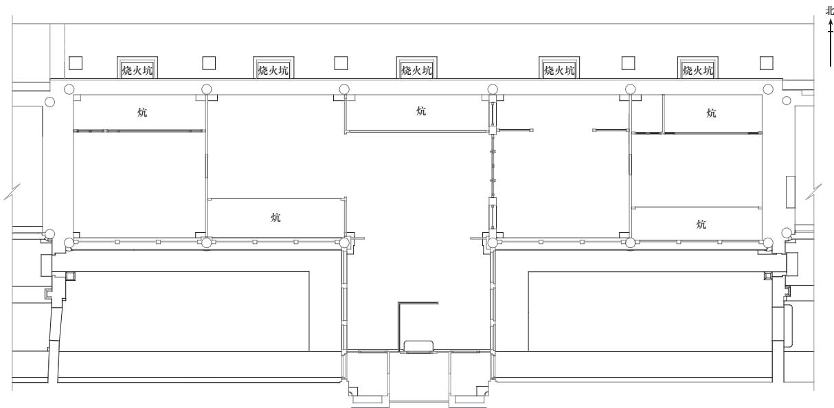
图17 养心殿后殿平面图
