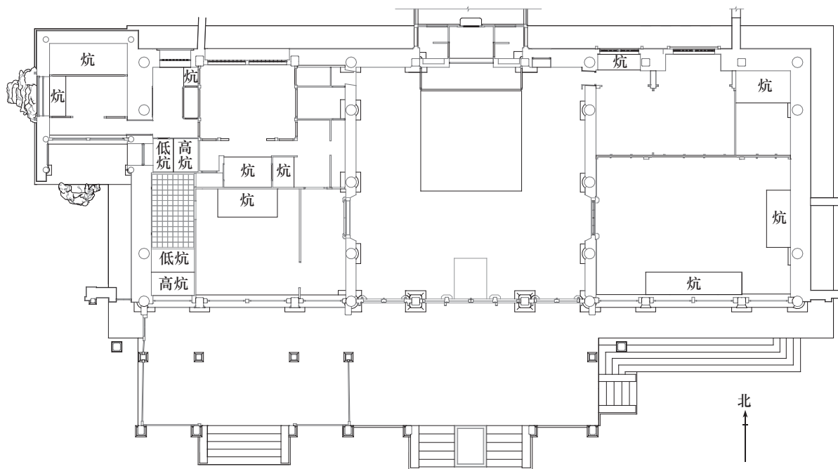
图3 养心殿平面图
