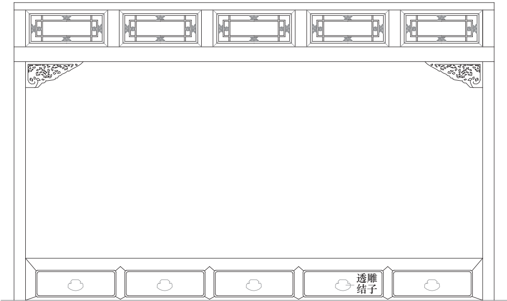
图57 几腿罩形式炕罩
