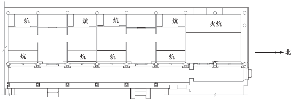
图46 西围房平面图
