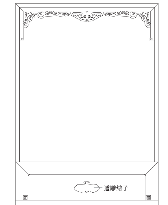
图62 几腿飞罩形式炕罩
