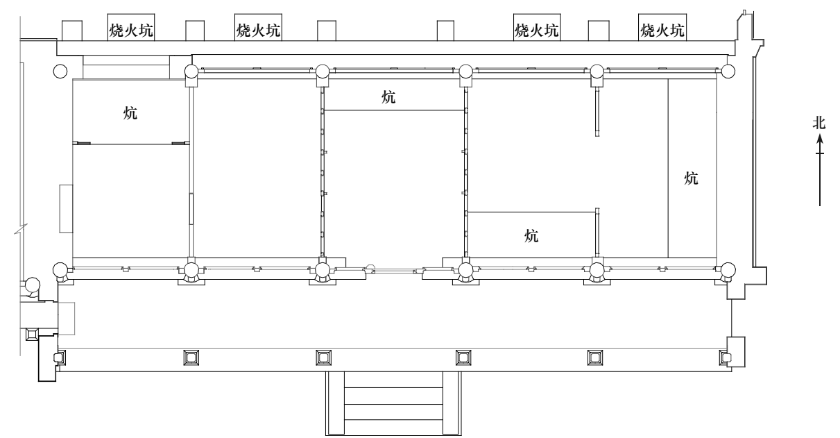
图23 体顺堂平面图
