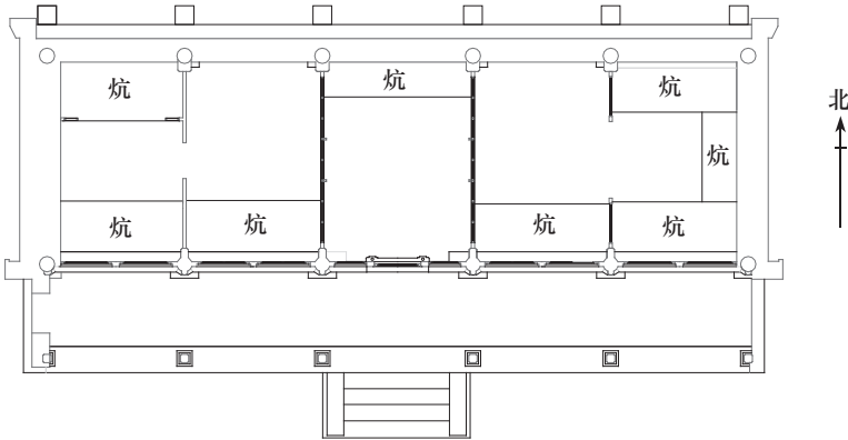
图28 燕禧堂平面图
