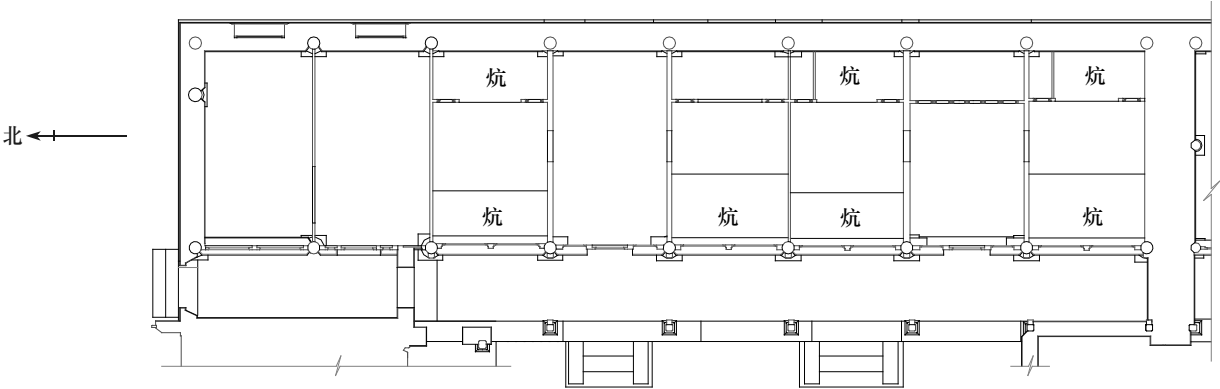
图38 东围房平面图
